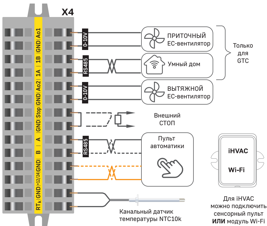
Рисунок 6 – Схема подключения малосигнальных цепей
